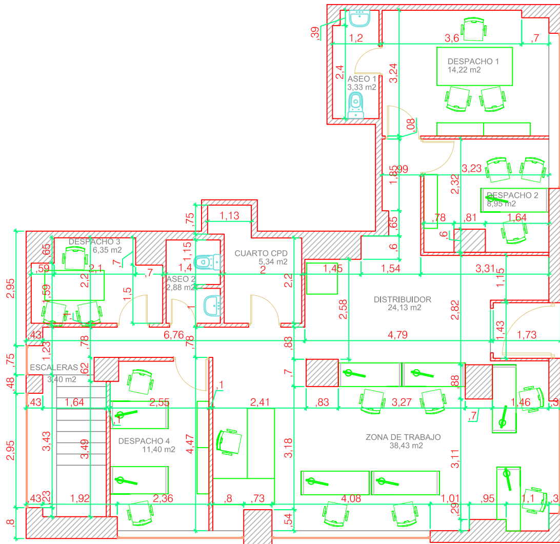
PLANTA BAJA ESTADO REFORMADO E 1:100
