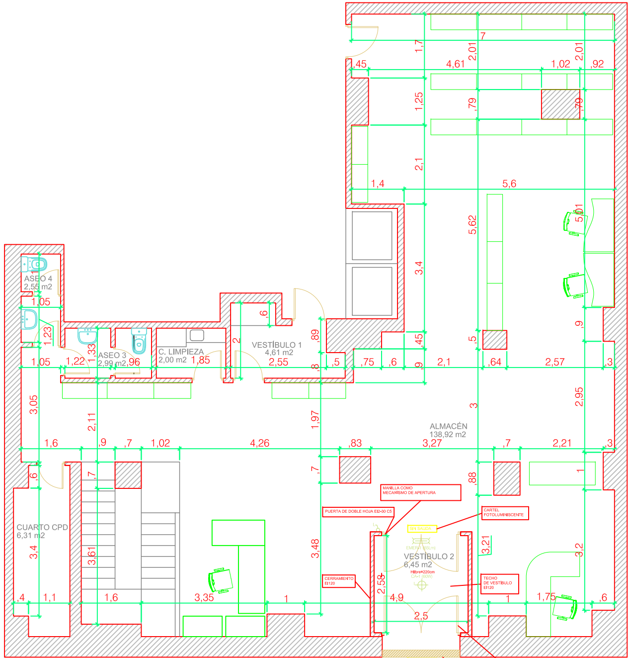
PLANTA SÓTANO ESTADO REFORMADO E 1:100
