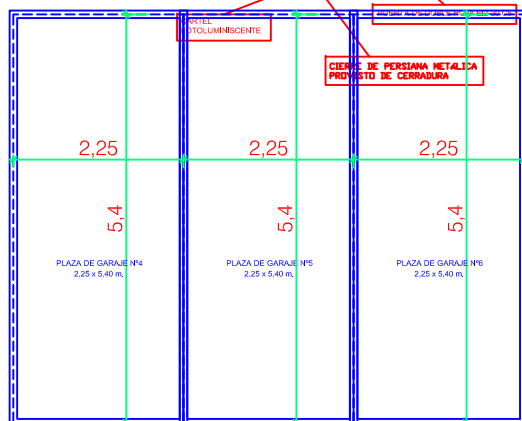
PLANTA SÓTANO ESTADO REFORMADO E 1:100
